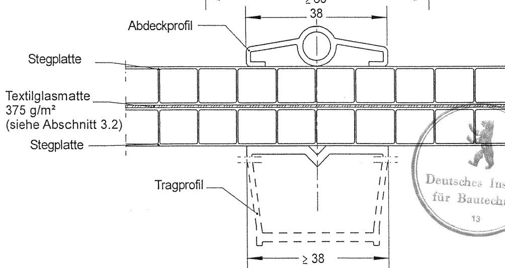
Schnitt C-C
