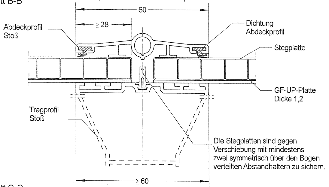
Schnitt C-C
