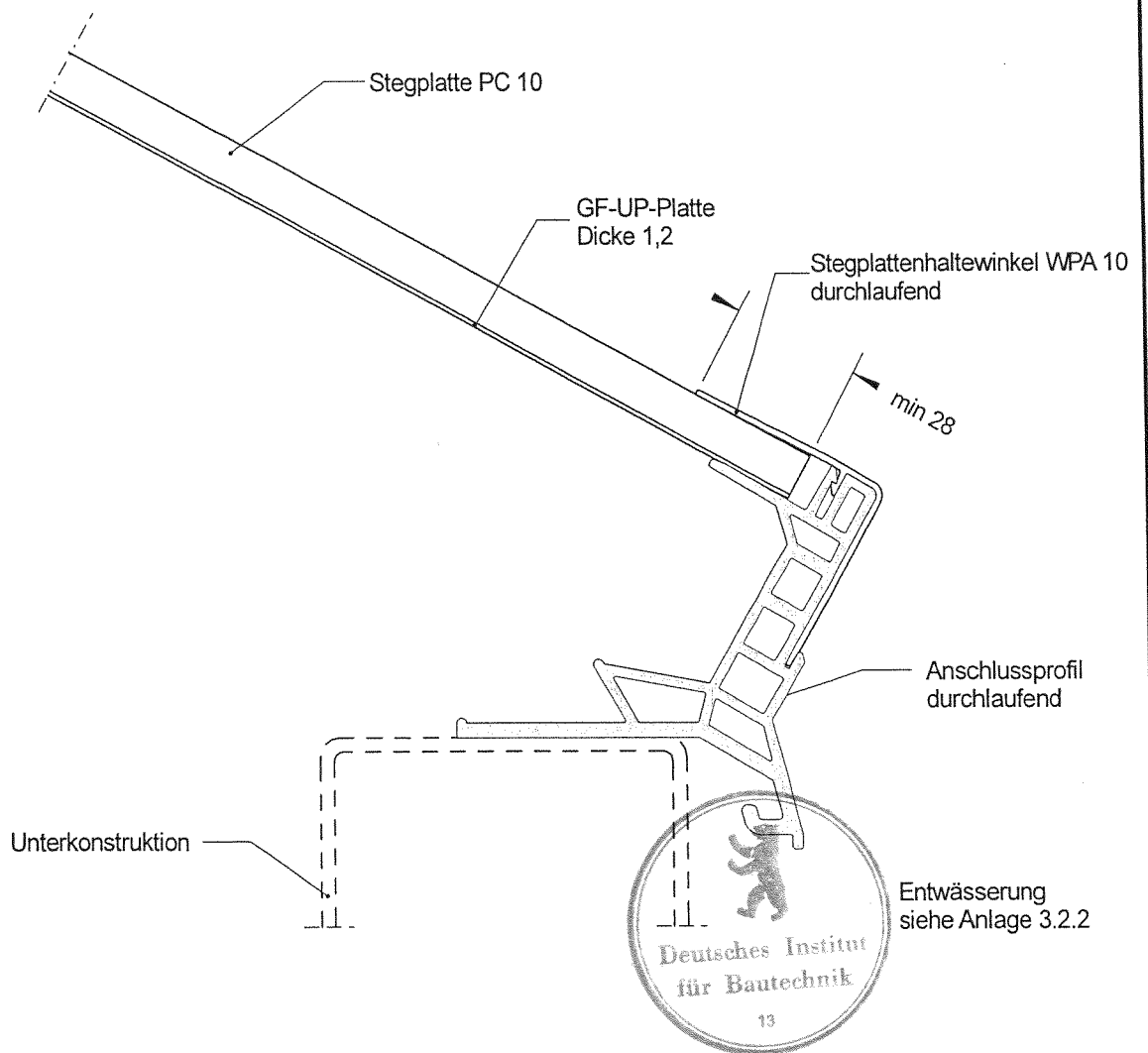
Stegplattendarstellung schematisch!
