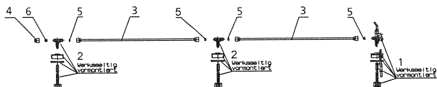
Entnahmeleitung
