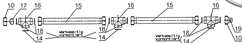
Entlüftungsleitung
