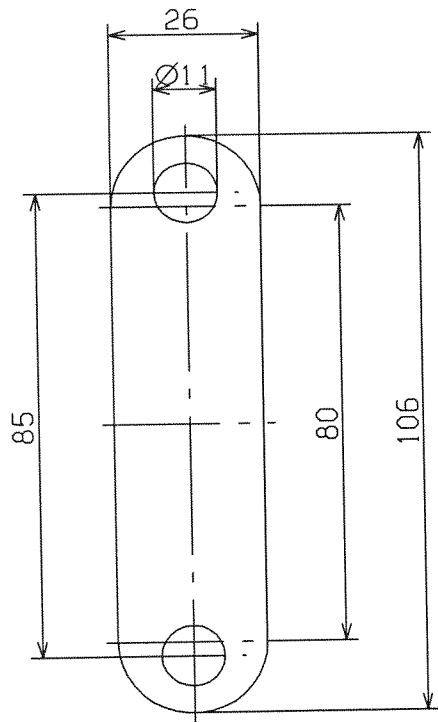
Abstandhalter
