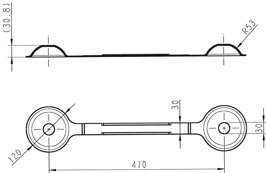
Schraubkappe Werkstoff: PE-HD
