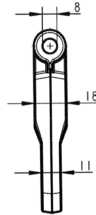
Griff für Behälter Werkstoff: PE-HD
