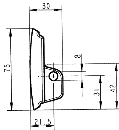
Einschlag-Griffplatte Werkstoff: PE-HD
