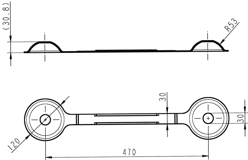
Schraubkappe Werkstoff: PE-HD
