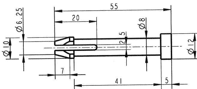
Bolzen für Griff Werkstoff: PE-HD
