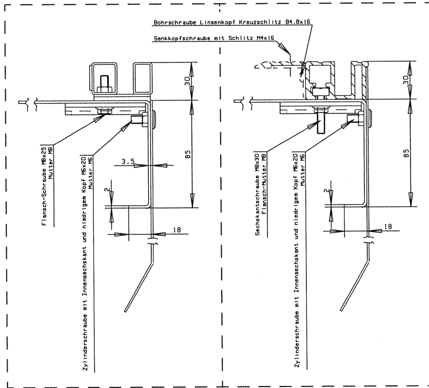
B) Stahlprofil
