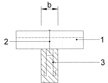
Bild 3 Beton- Auflager
