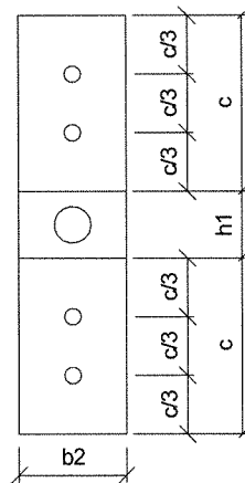
hinteres Blech - t 2
