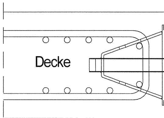
Bewehrungsführung s. Detail Anschluss Platte / Platte
