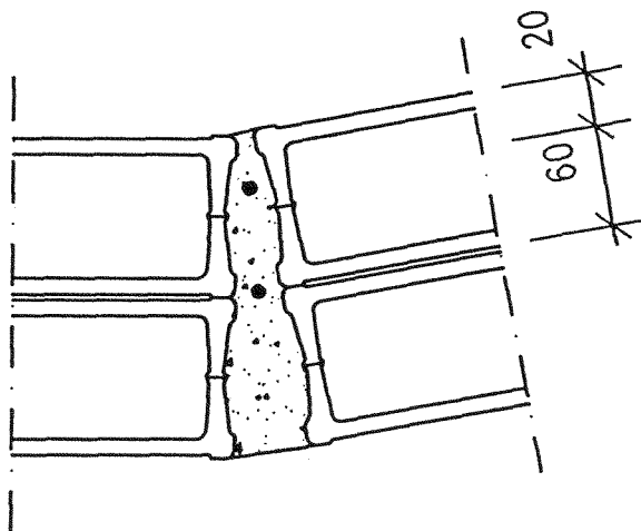
Fuge mit Lage der Bewehrung
