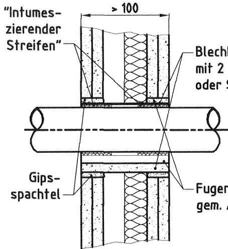
Einbau von Blechhülsen oder Halbschalen
