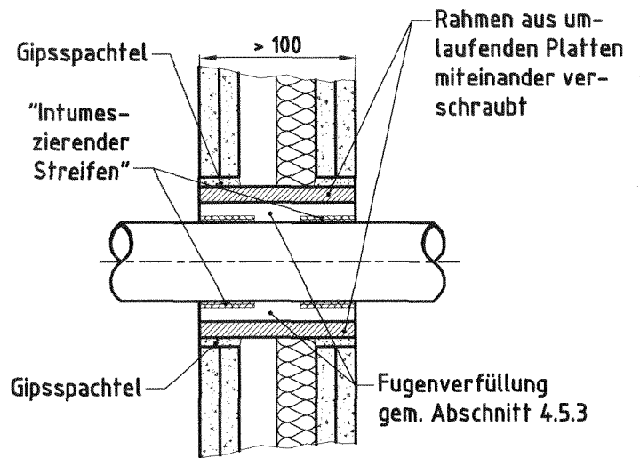
Einbau von Rahmen (Platten verschraubt)
