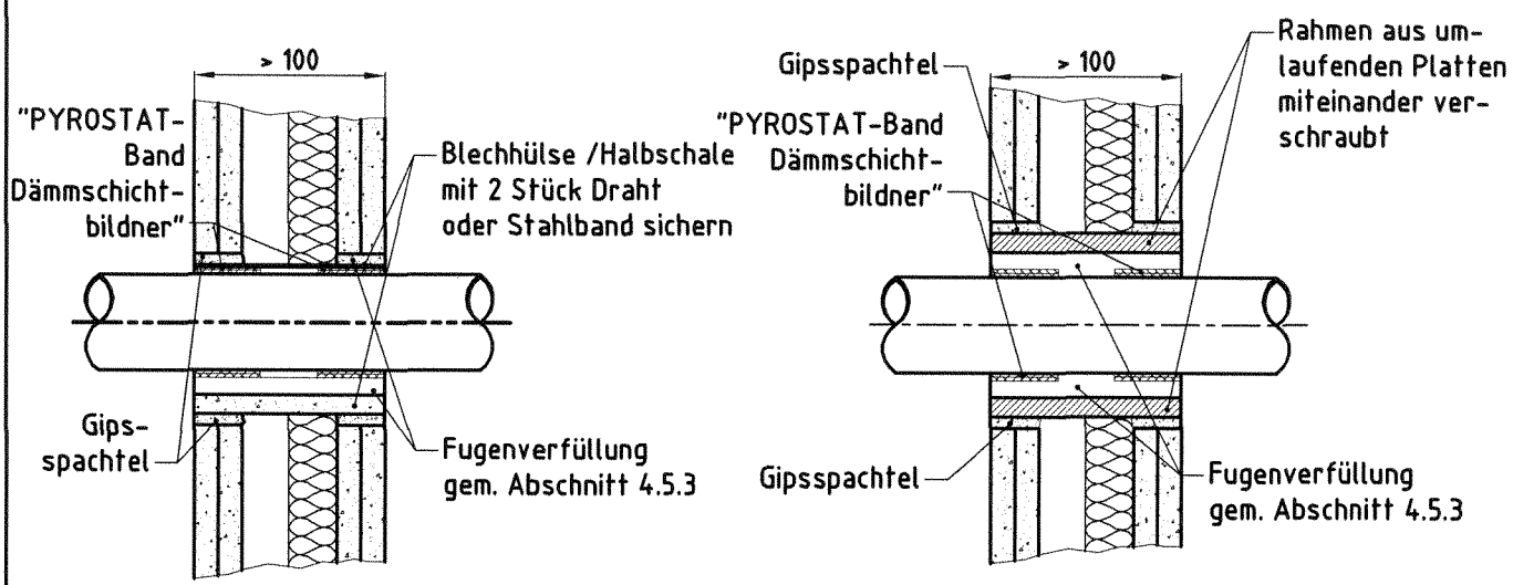
Einbau von Blechhülsen oder Halbschalen
