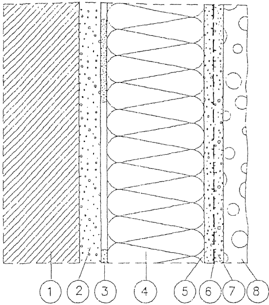
Geklebttes WDVS
