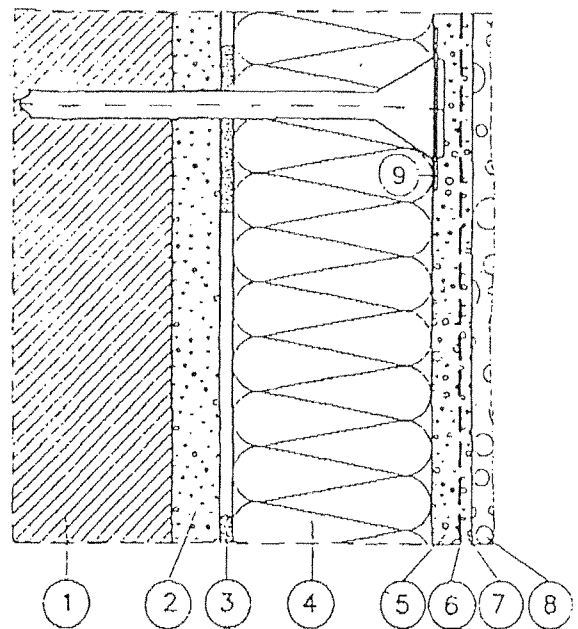
Mit Dübeln mechanisch befestigtes WDVS und zusätzlichem Klebemörtel
