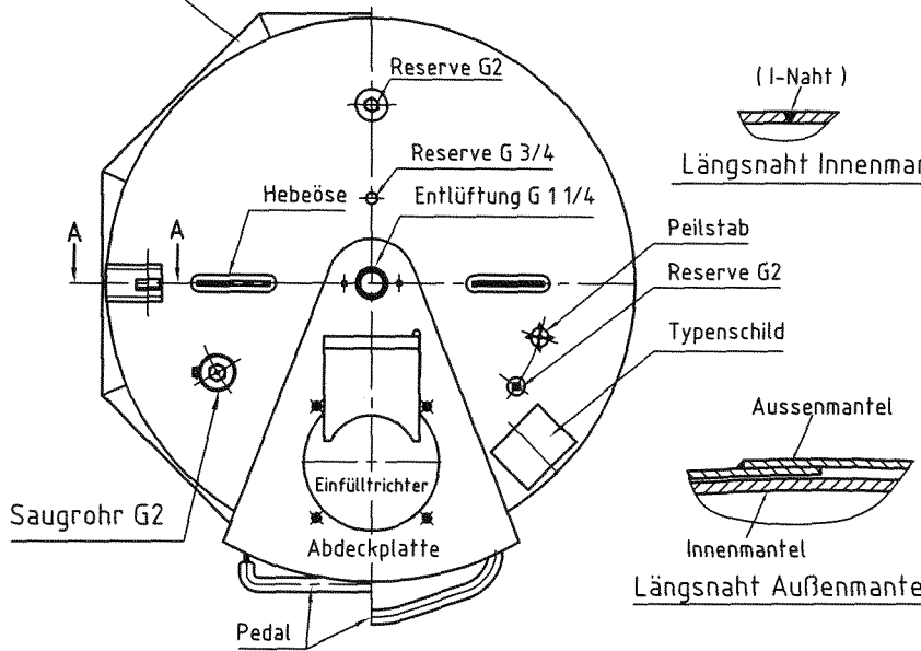
Behälterausführung GD 250 siehe Zeichnung PB 3915-2
