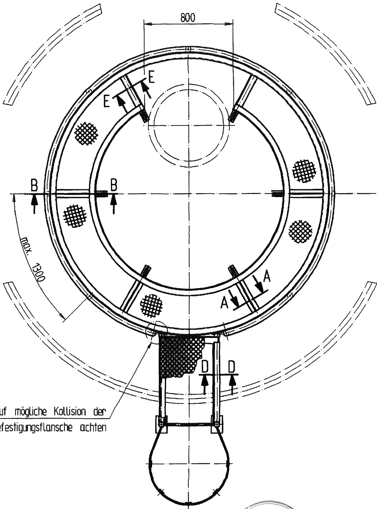
Draufsicht Gitterbühne 90° gedreht
