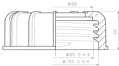
Überwurfmutter
