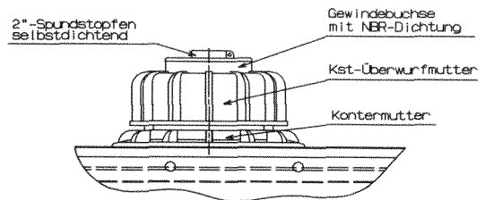
Detail Y
