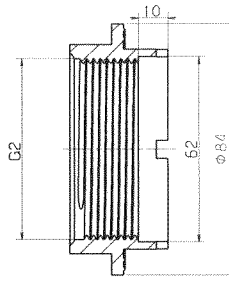
Stopfen
