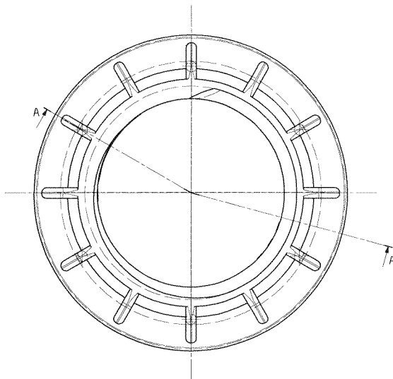
Kontermutter
