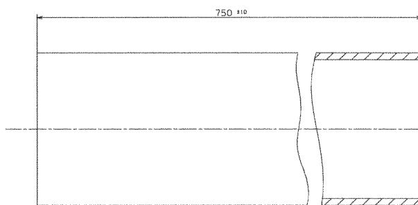
Einsteckrohr
