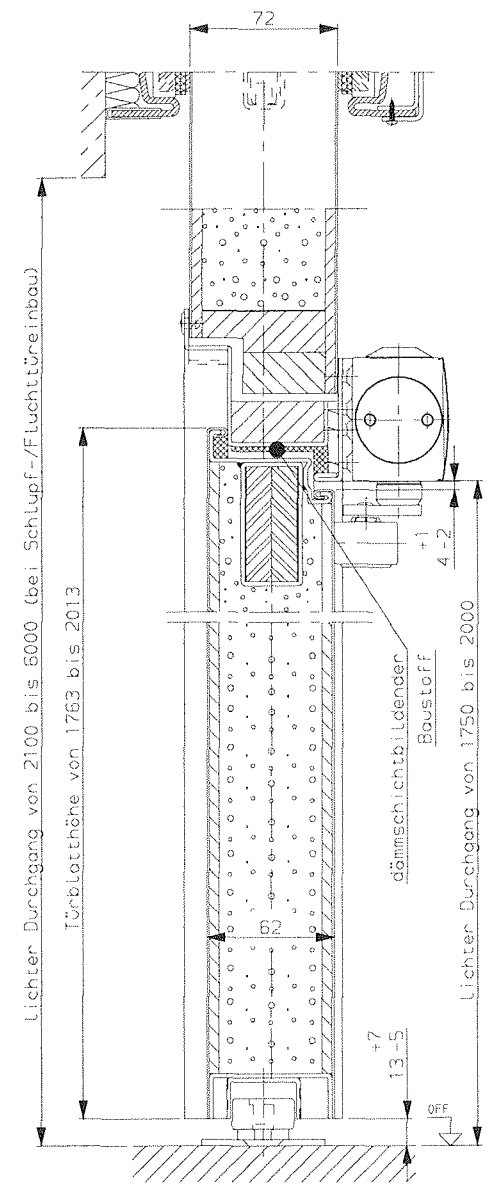
Schnitt B-B
