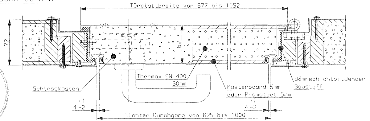
Schnitt A-A
