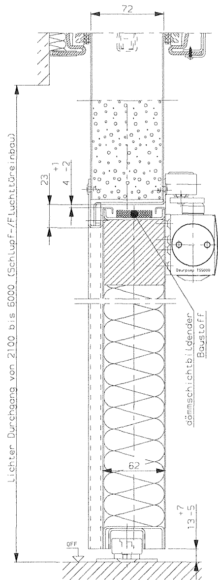
Schnitt B-B
