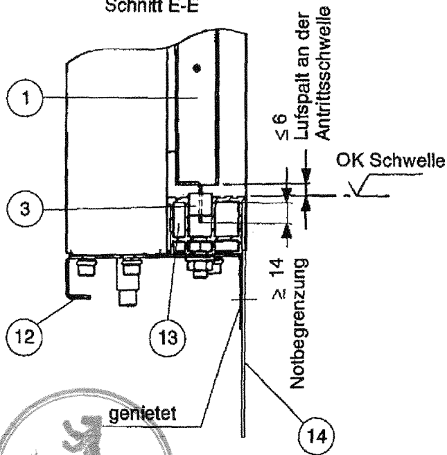
Schnitt E-E
