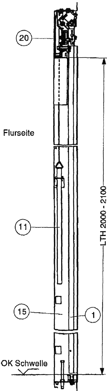
Schnitt C-C
