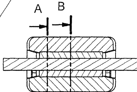
Schnitt C-C M 1:1
