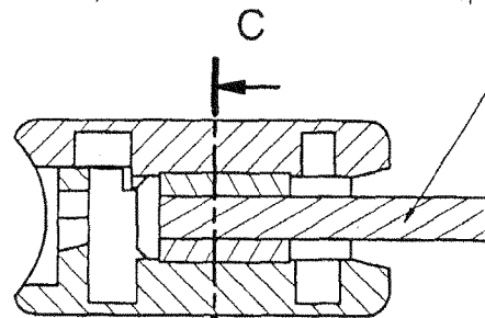
Schnitt B-B M 1:1
