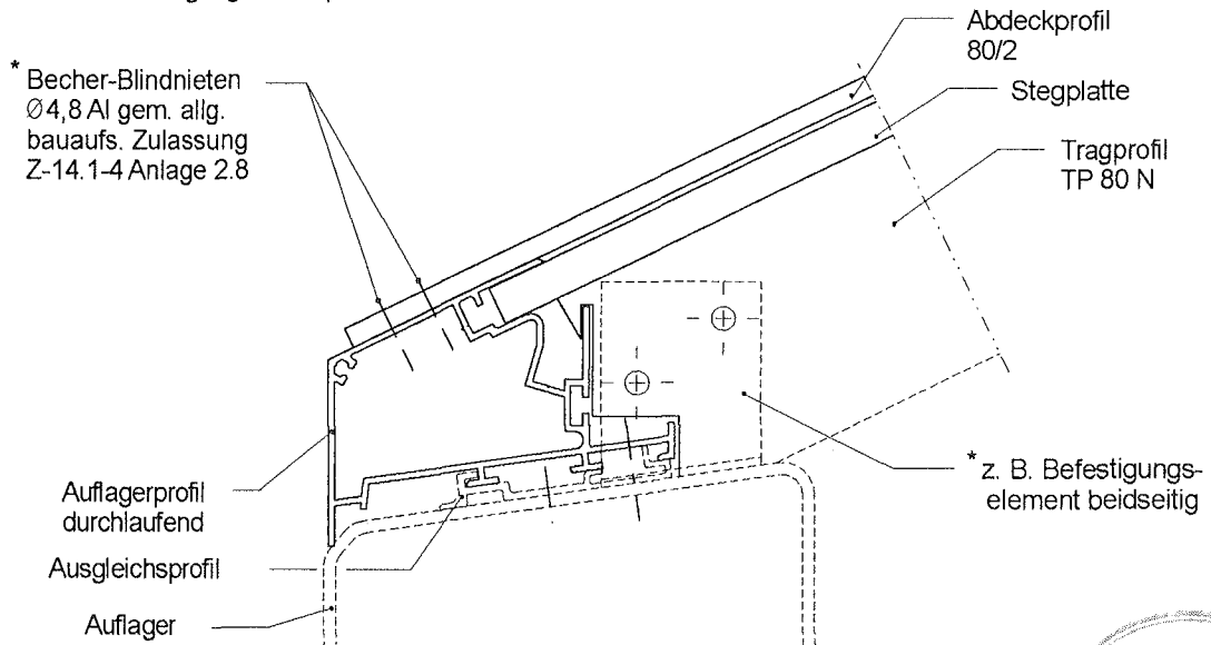
alternative Befestigung Abdeckprofil
