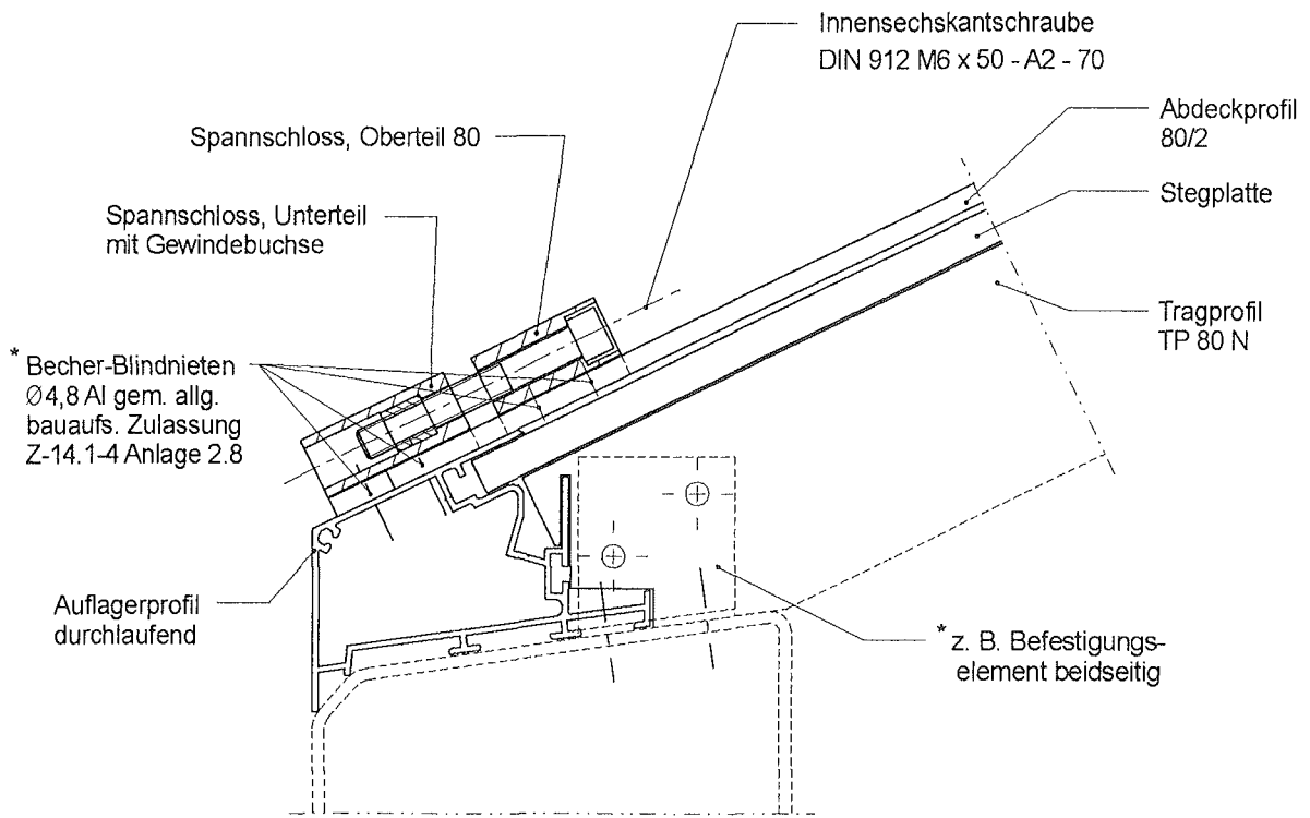
alternative Befestigung Abdeckprofil
