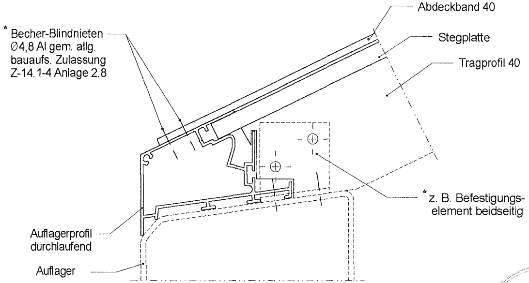
alternative Befestigung Abdeckband
