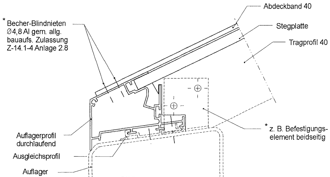
alternative Befestigung Abdeckband
