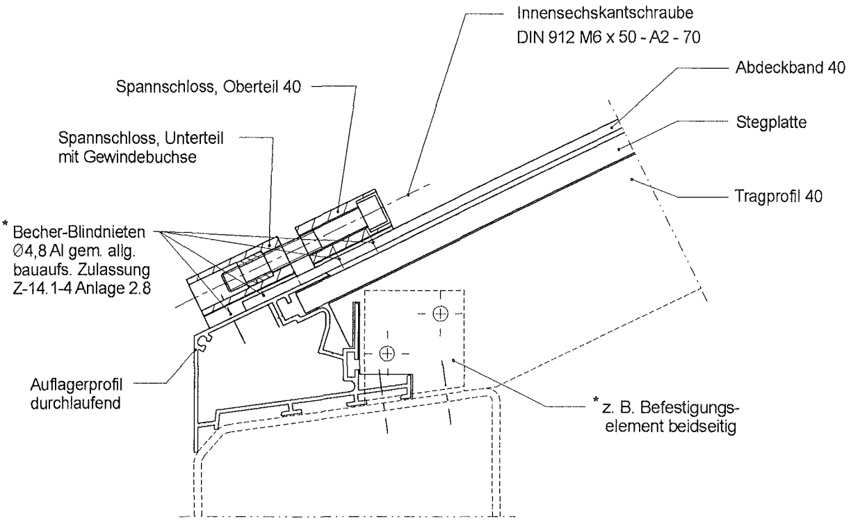
alternative Befestigung Abdeckband
