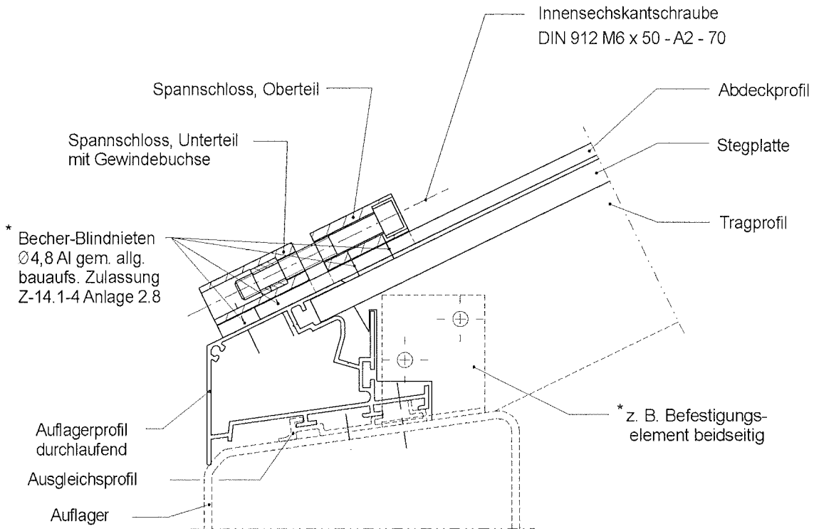
alternative Befestigung Abdeckprofil
