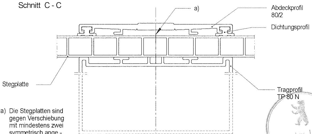
Stegplattendarstellung schematisch!
