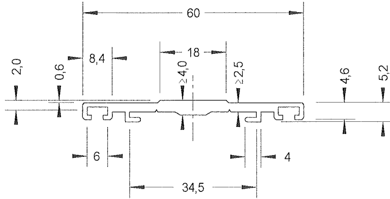
Abdeckprofil 60/2
