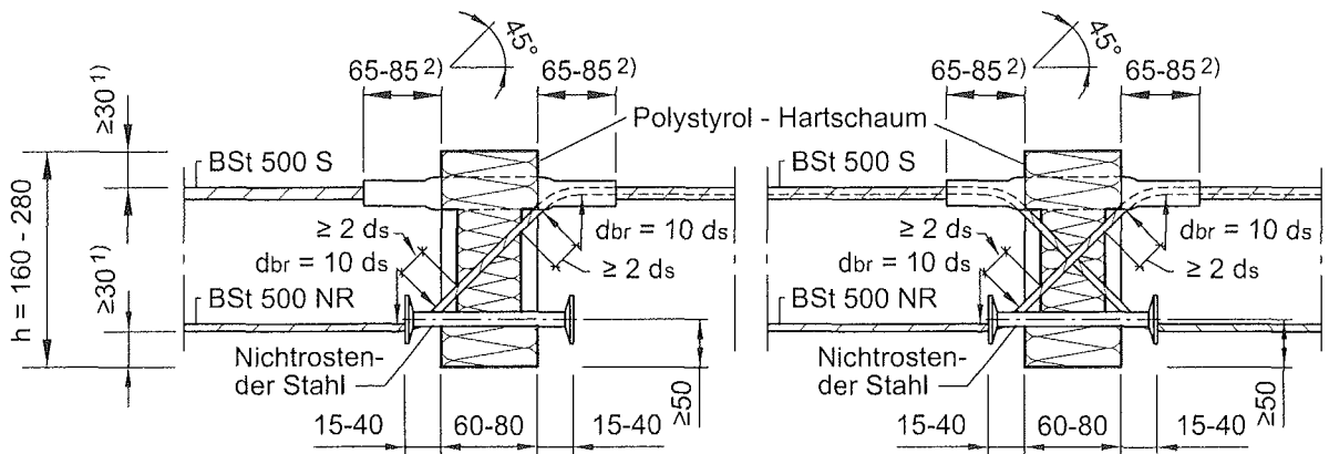
Abb. 13: Typ HIT-BX
