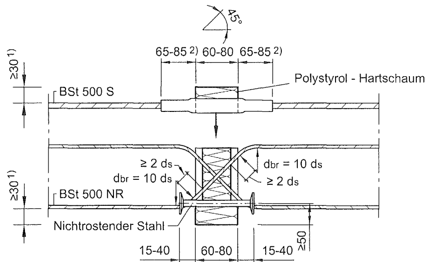
Abb. 17: Typ HIT-BF-±Q
