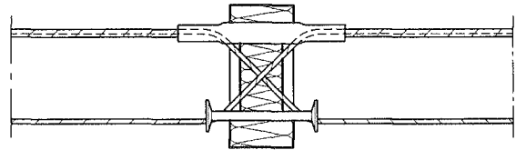
Abb. 2: Halfen - Iso - Element Typ HIT-BX-±Q
