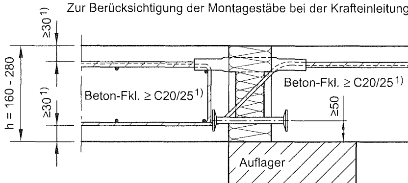
Abb. 16: Beispiel Halfen - Iso - Element Typ HIT-BX mit Aufhängebewehrung
