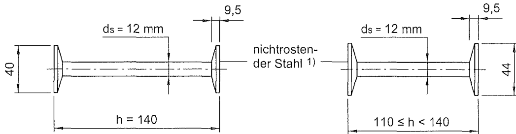
Abb. 12: Doppelkopf-Drucklager 2) aus nichtrostendem Stahl
