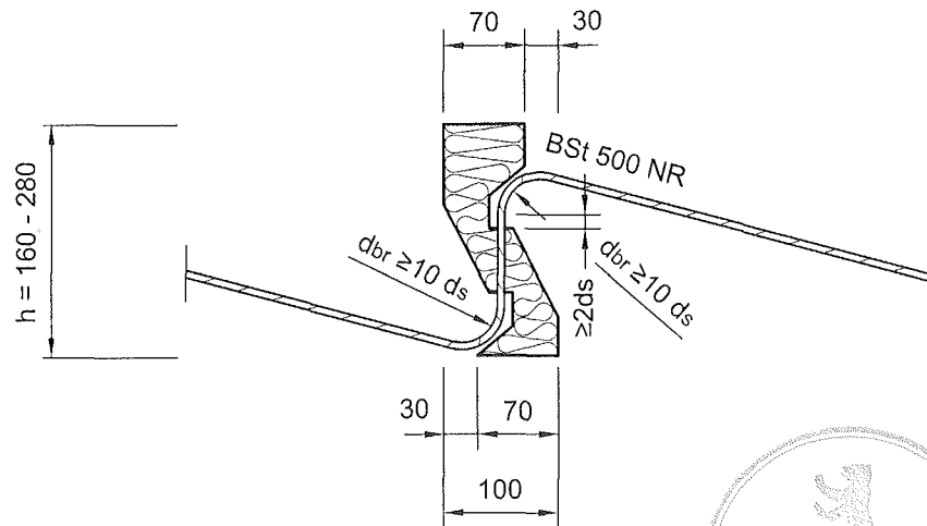
Abb. 22 Halfen-Iso-Element Typ HIT-VT
