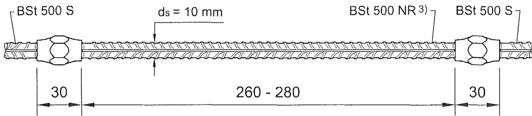
Abb. 9: Zugstab mit Verpressmuffe
