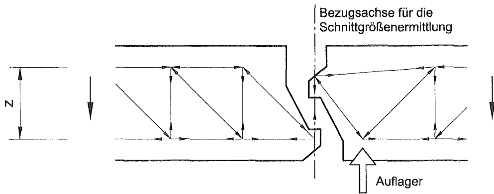
Abb. 29: Typ HIT-VT
