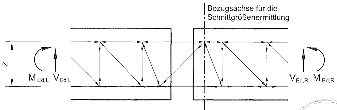
Abb. 28: Typ HIT-BD, HIT-BDR ( V_{Ed,L} < V_{Ed,R} )
