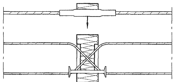
Abb. 4: Halfen - Iso - Element Typ HIT-BF-±Q
