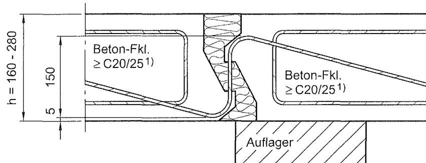
Abb. 23 Halfen-Iso-Element Typ HIT-VT mit Aufhängebewehrung
