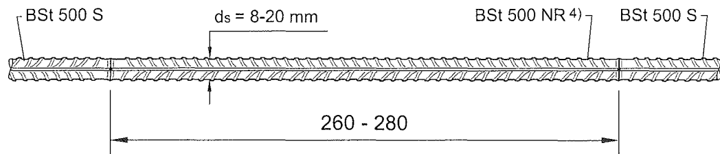
Abb. 11: Zugstab mit geschweißten Stößen
