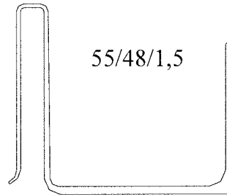
Profil-Nr.: 962/1 für einschalige Verglasung
