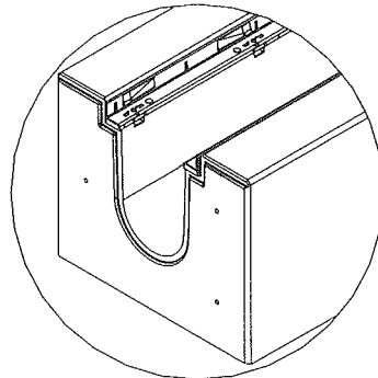
ohne Stahlblechabdeckung
