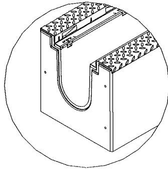
mit Stahlblechabdeckung
