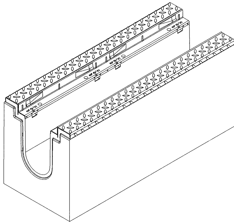
mit Stahlblechabdeckung
