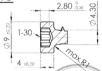
SCHNITT D-D MABSTAB (2:1)
