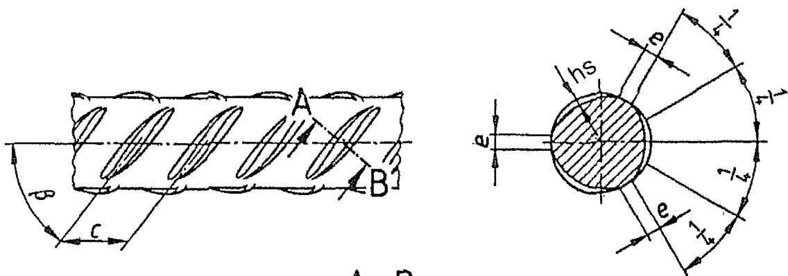
Schnitt A - B (vergrößert)
