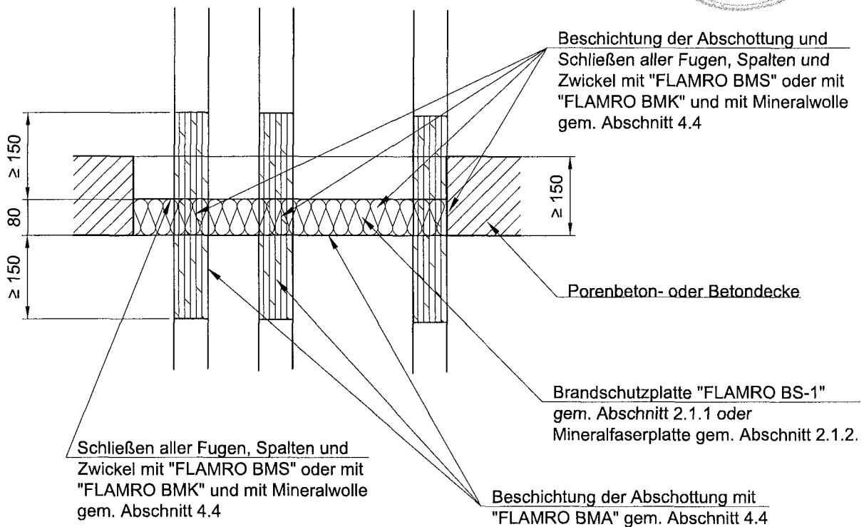
Schnitt
