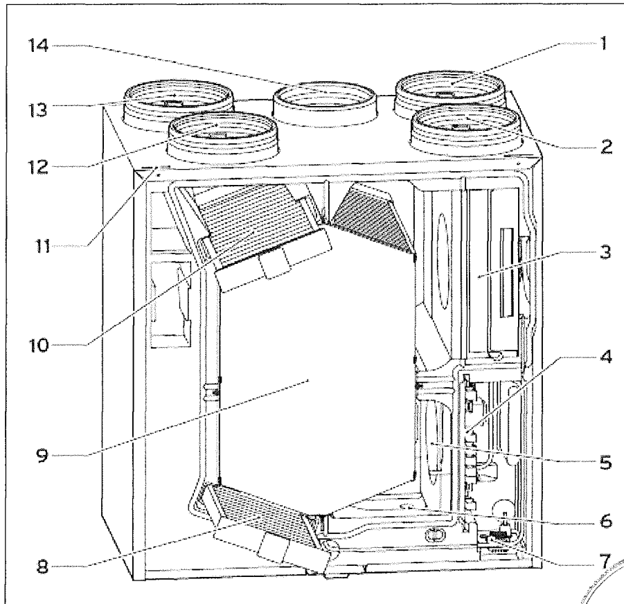
Abb. 4.2 Aufbau recoVAIR VAR 350
