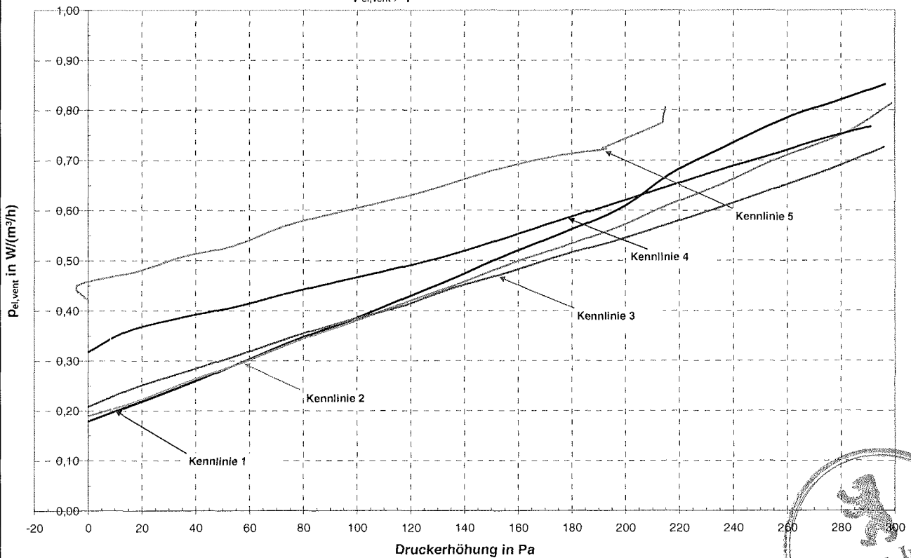
P_{el,vent}, \Delta p -Kennlinien Abluft/Fortluft
