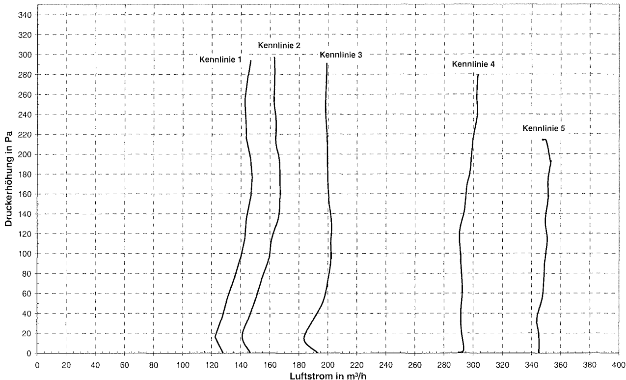
\Delta p, \dot{V} -Kennlinien Außenluft-/Zulufttrakt
