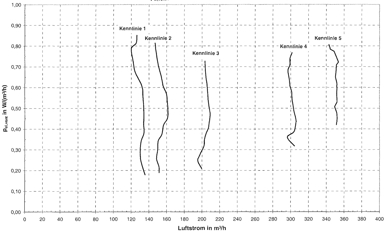
P_{el,vent}, \dot{V} -Kennlinien Abluft/Fortluft
