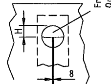
Schnitt A-A für NS 10 ( \phi 1200 ) u. NS 10 + 15 ( \phi 2000 ) u. NS 20 ( \phi 2000 ) Freier Querschnitt
