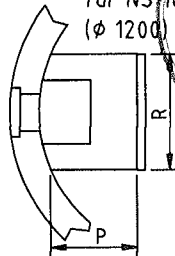
Zulaufdetail für NS/10 ( \phi 1200 )
