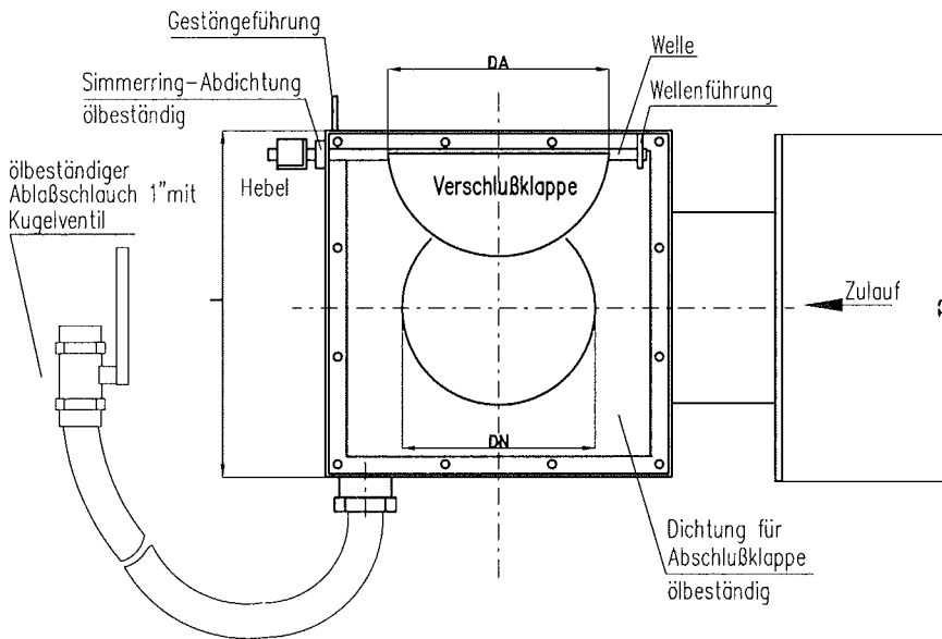
Horizontalschnitt
