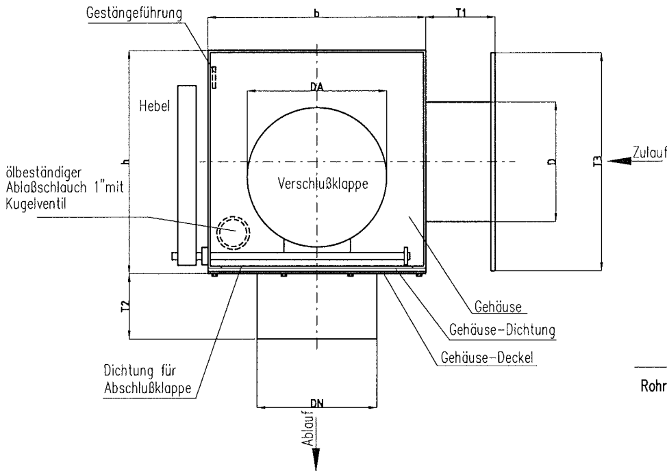
Horizontalschnitt
