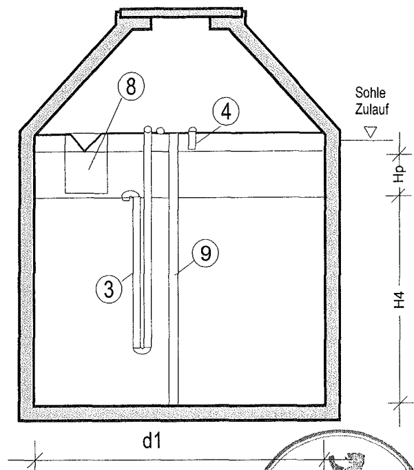
Schnitt B-B
