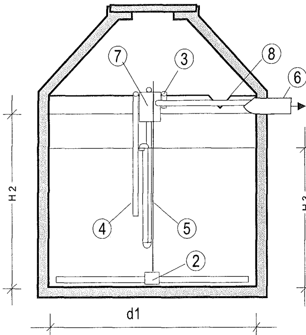
Schnitt A-A
