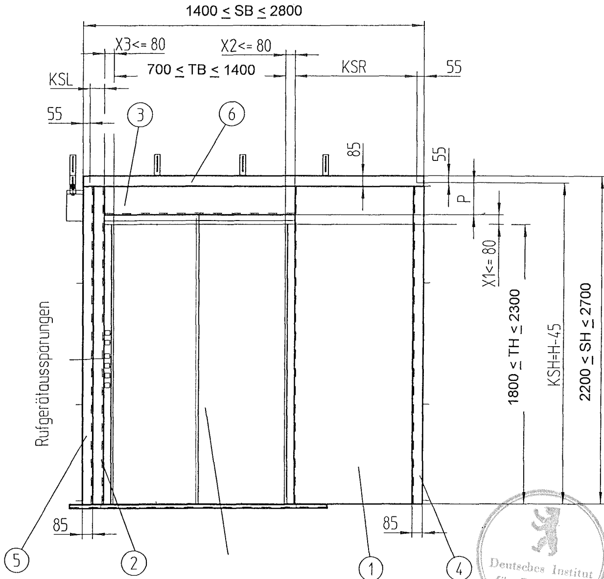
Fahrschacht-Teleskop-Schiebetür "Typ LD 2T" der Fa. Haushahn siehe Anlagen 5, 6, 9, 10, 11
