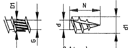
Optional: Bohrspitze mit Schneidkerbe
