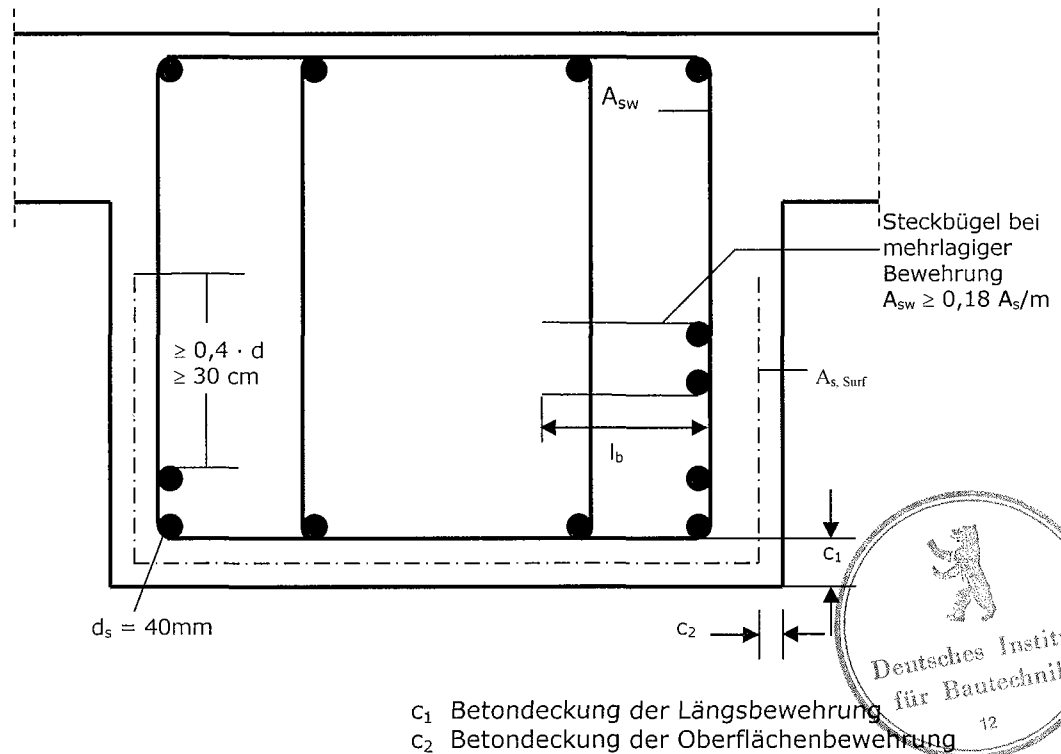
Bild 4b Balken und Anordnung von Steckbügeln bei mehrlagiger Bewehrung
