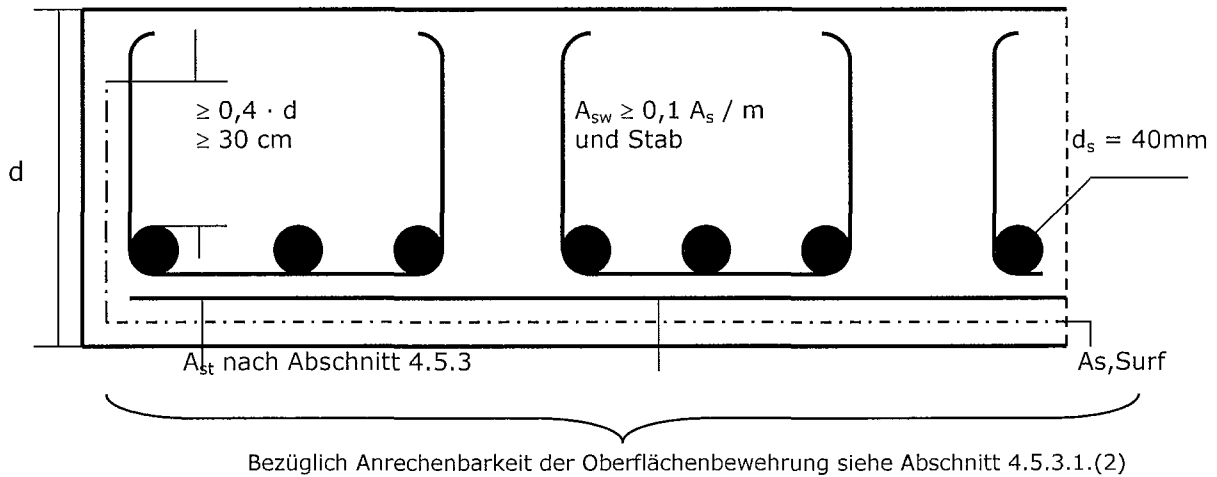
Bild 4b Balken und Anordnung von Steckbügeln bei mehrlagiger Bewehrung
