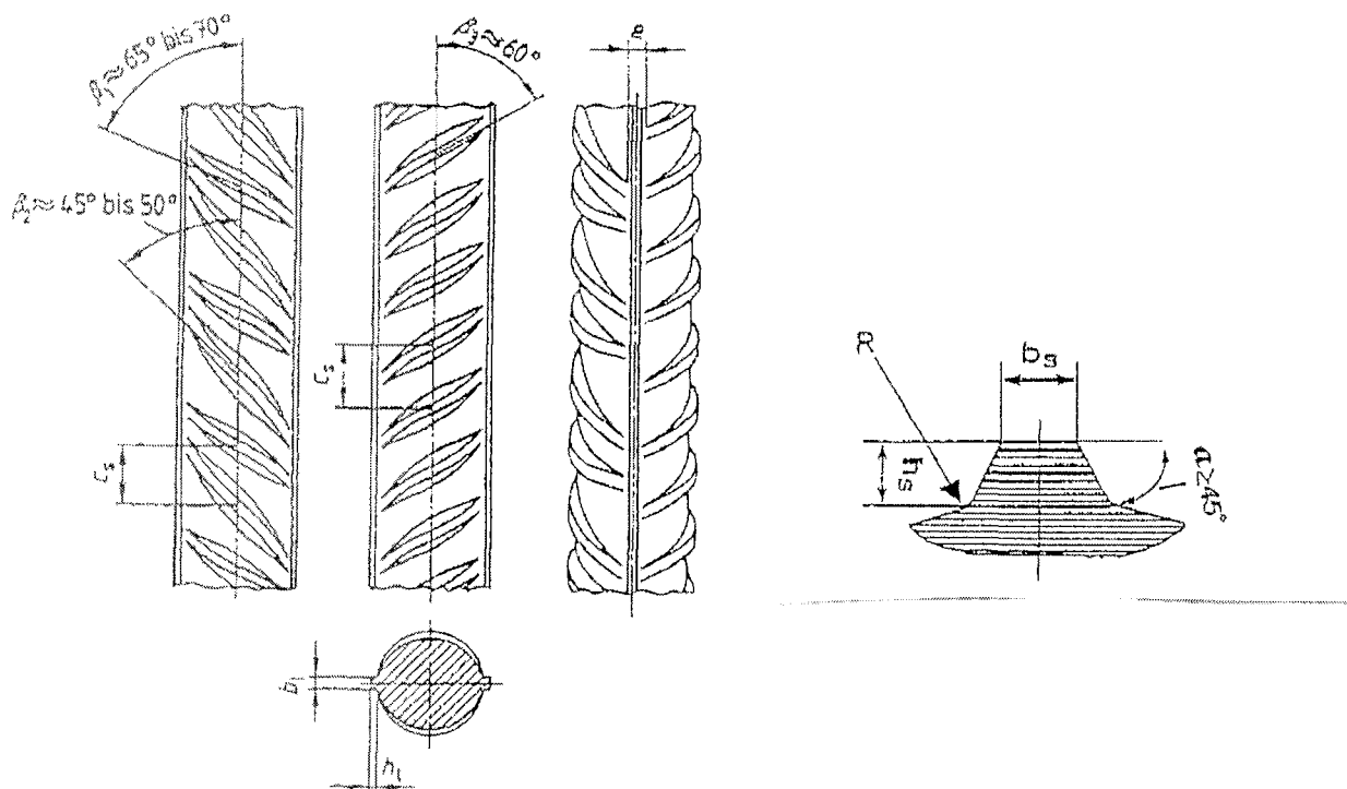
Schrägrippen, Querschnitt in Rippenmitte Ausrundungsradius R \geq 2,5\text{mm}
