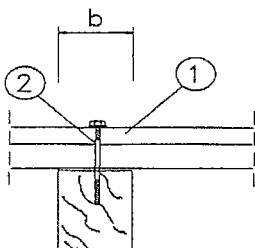
Holz-Auflager
