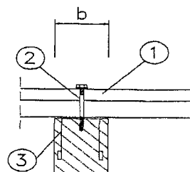
Beton-Auflager
