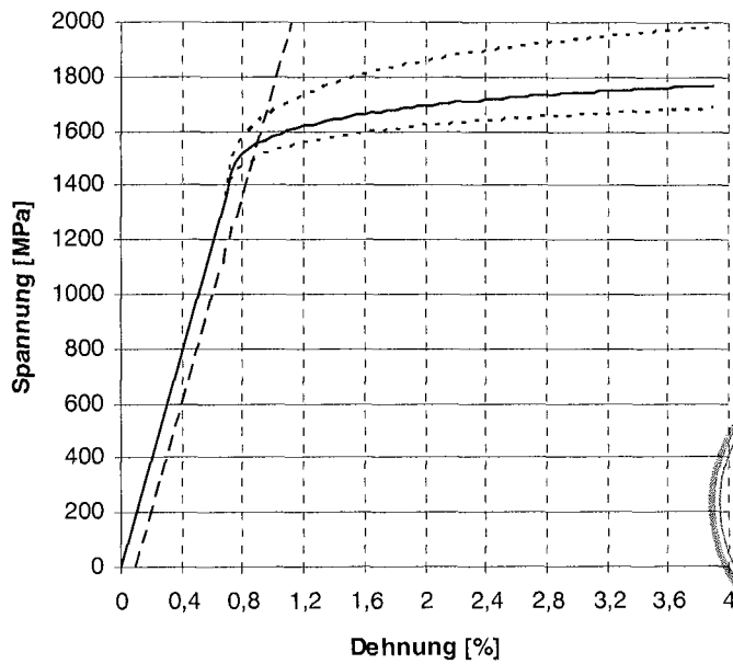
Bild 2: Spannungs-Dehnungslinie
