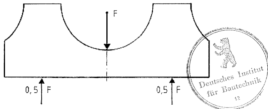
Bild 1: Belastungsanordnung Biegeversuch
