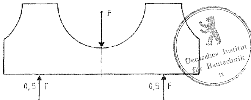
Bild 1: Belastungsanordnung Biegeversuch
