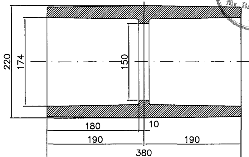
Muffe für Pfähle Ø 170
