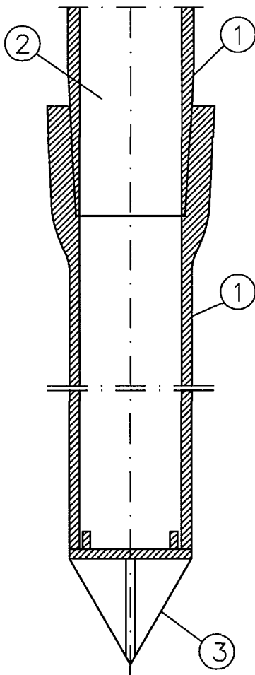
Pfahlfuß, Typ A
