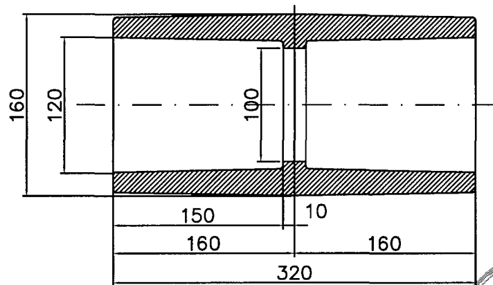
Muffe für Pfähle Ø 118
