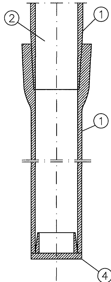
Pfahlfuß, Typ B
