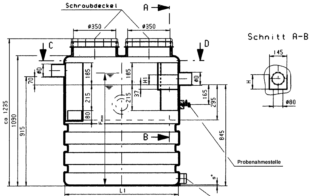
Schnitt C-D
