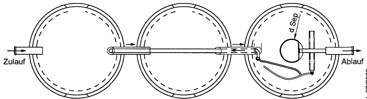
Grobfang / Schlamm-speicher
