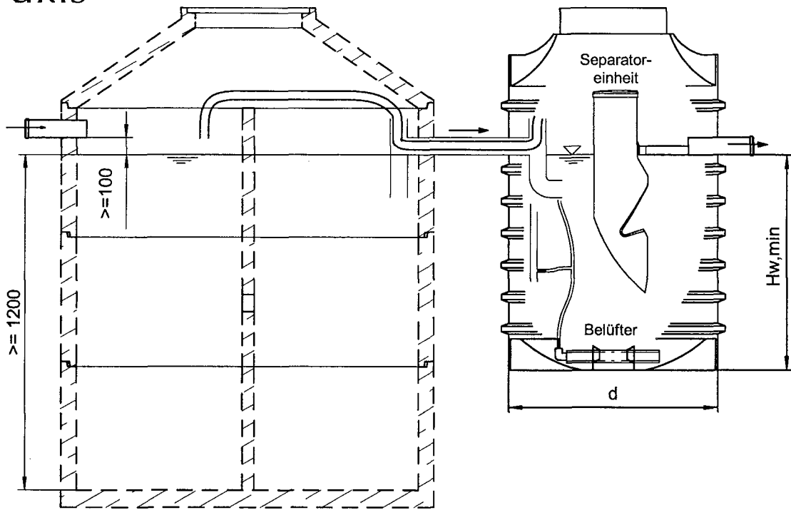
Grobfang / Schlamm-speicher (vorhanden)
