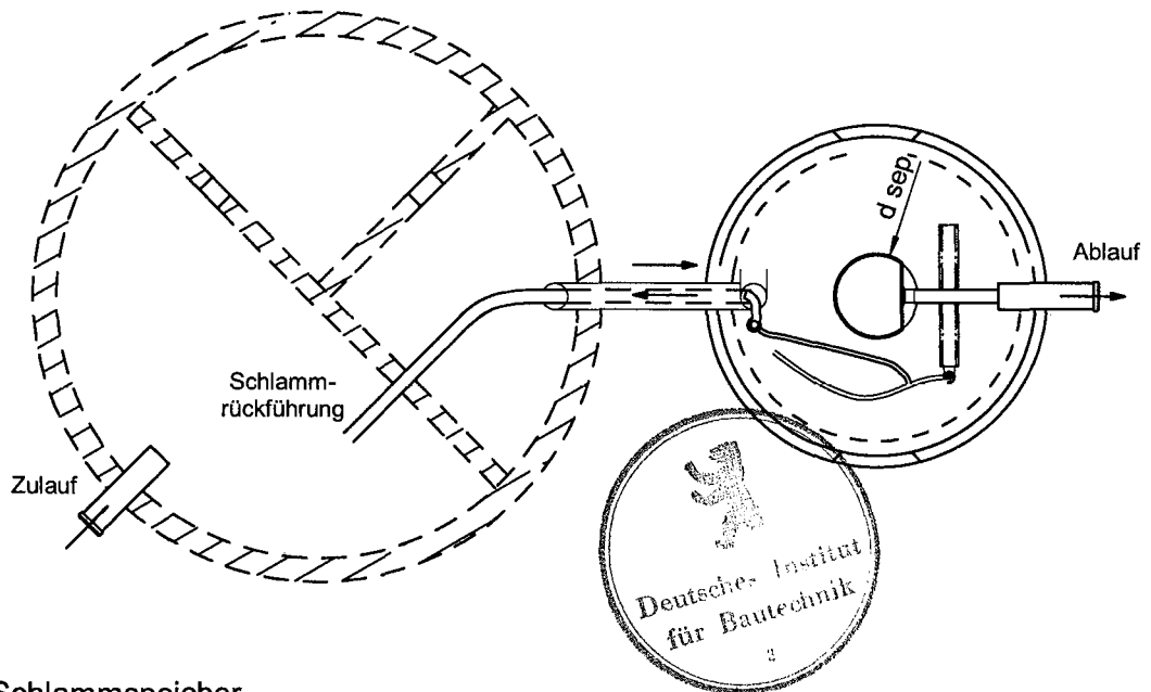
Grobfang / Schlamm-speicher (vorhanden)
