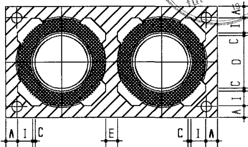
Schornsteingruppe
