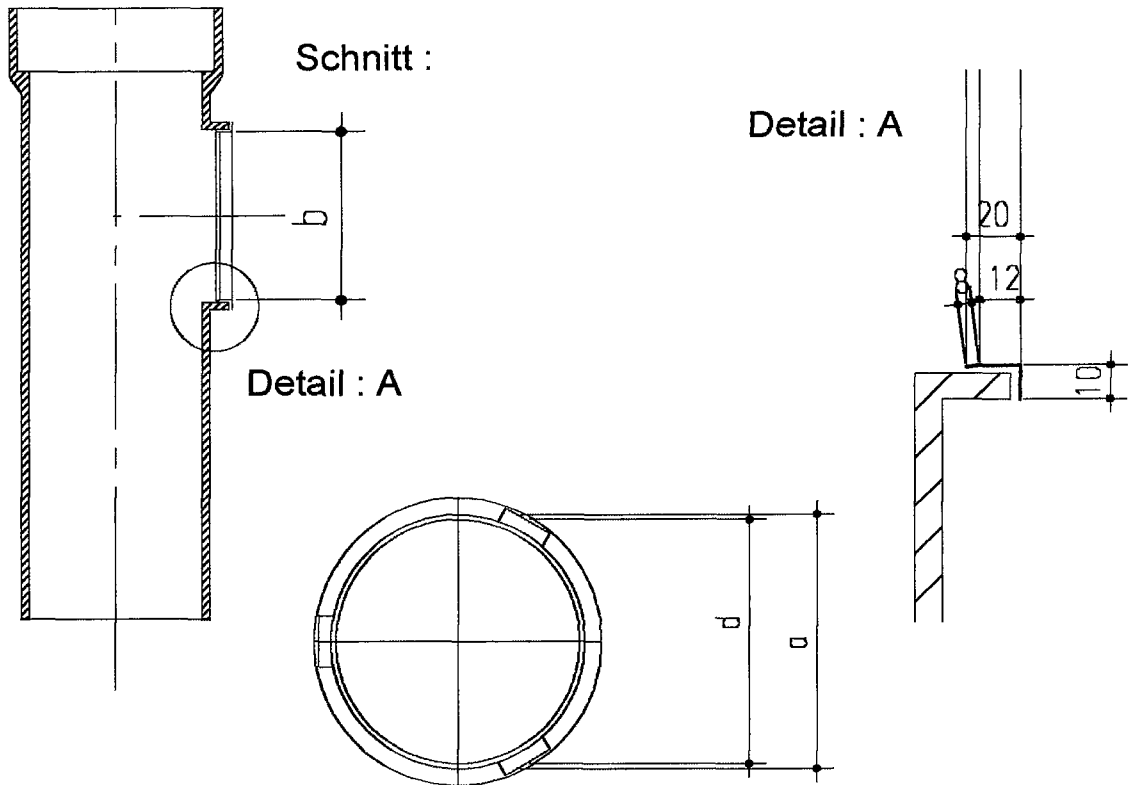
Draufsicht
