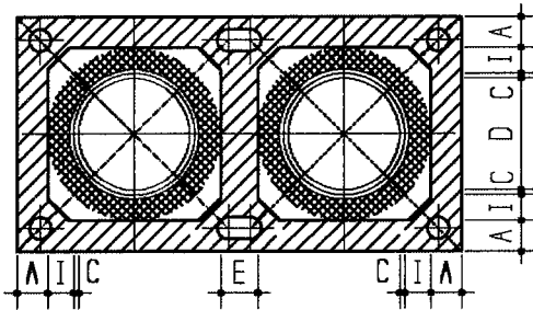
Schornsteingruppe
