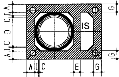
Einzelschornstein mit Schacht
