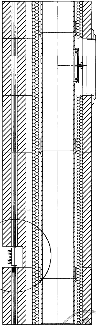
Schnitt : A - A
