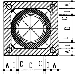
Einzelschornstein
