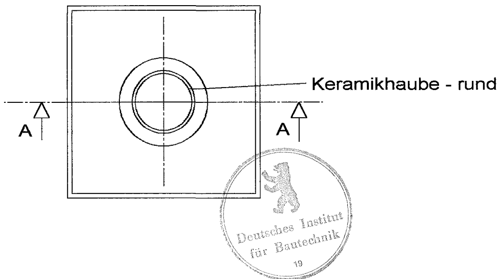
Draufsicht
