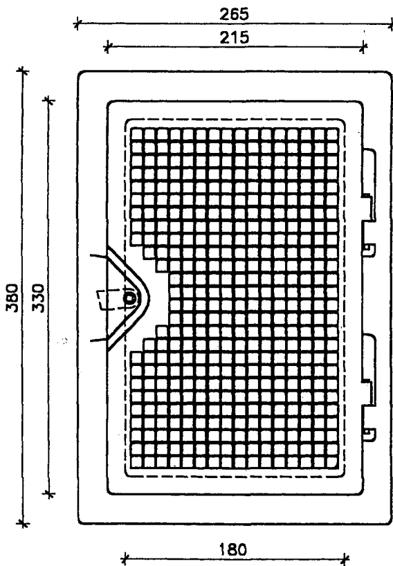
Gittertür mit Lochgröße 10 x 10 mm Materialdicke 1mm
