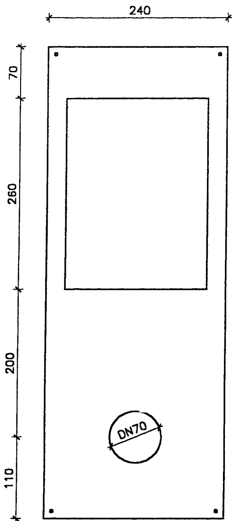
Blende Abkantung 1cm, umlaufend Material ST 37, verzinkt, pulverbeschichtet
