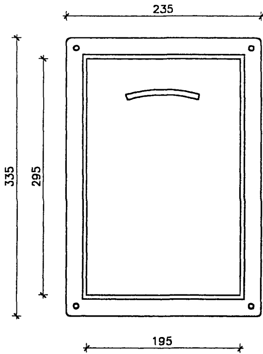
Reinigungstür mit einhängbarer Innentür Materialdicke 0,7mm
