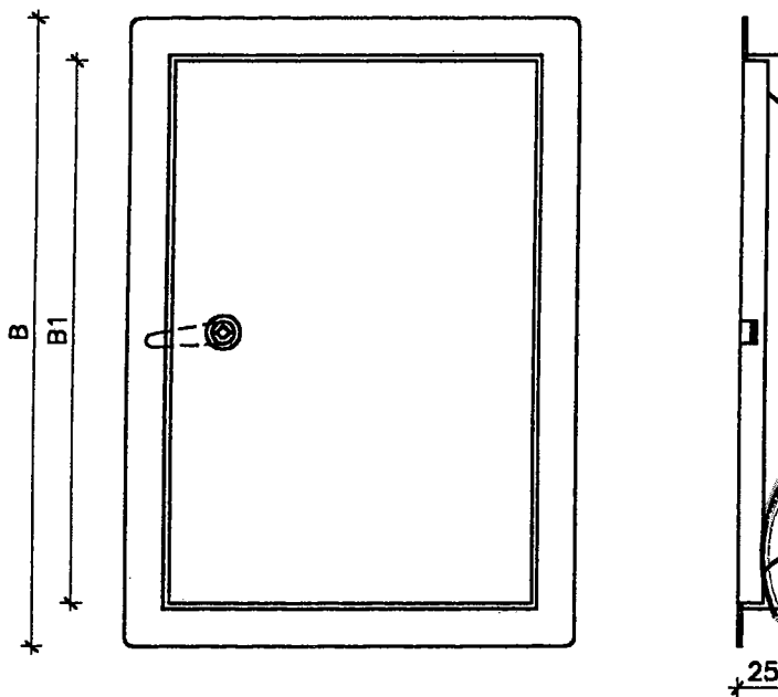
Reinigungstür mit geschlossenem / geschlitztem Türblatt
