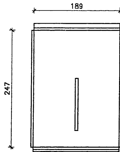
Einhängetür Material ST 37, verzinkt, pulverbeschichtet
