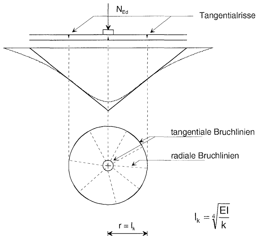
Bild 3: Statisches System zum Nachweis der Sohlplatten unter Einzellasten
