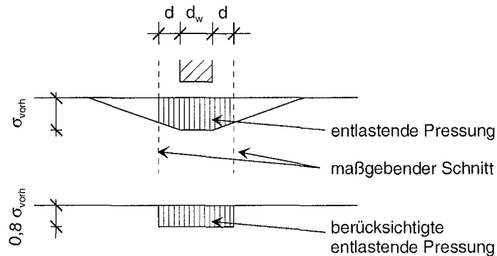
Bild 2: Entlastende Wirkung der Sohlspannung
