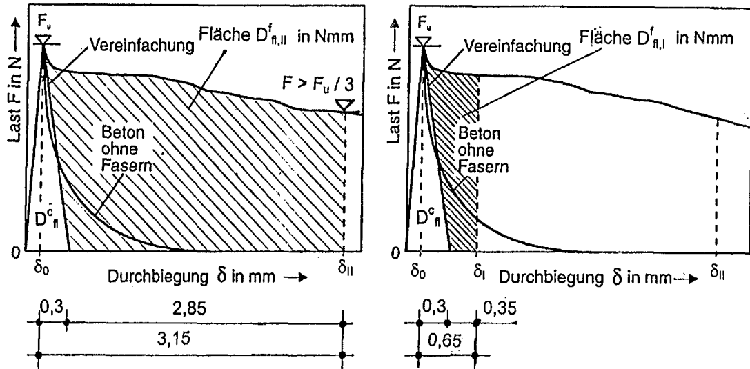
Bild 2. Ermittlung der äquivalenten Biegezugfestigkeiten f_{eq,I} bzw. f_{eq,II}
