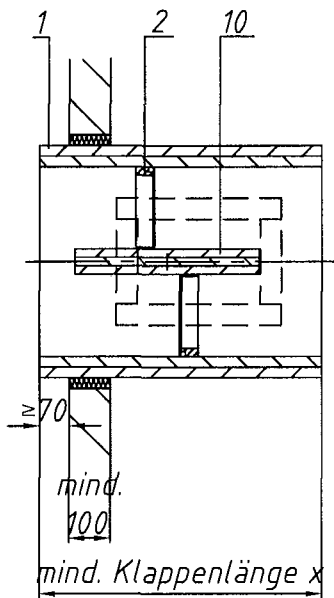
Darstellung ohne Anschlußprofil für Entrauchungsleitung 600° (Stahlblech)
