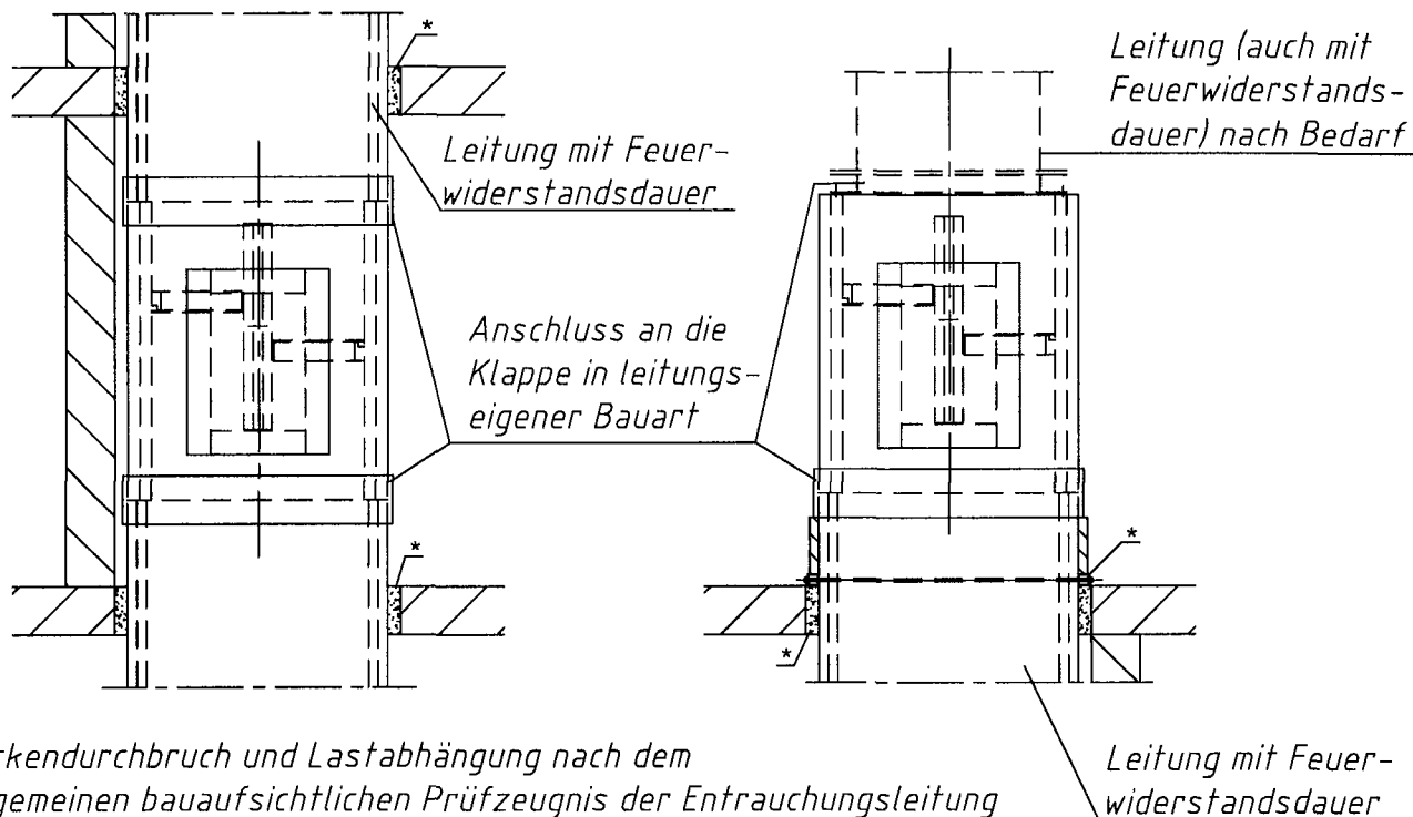
Darstellung des Anschlußprofils für Entrauchungsleitung 600° (Stahlblech)
