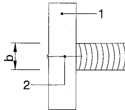
Bild 2 Holz- Auflager
