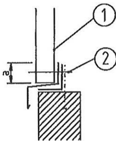
Bild 4 Fußpunkt Wandelement aufgesetzt
