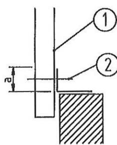
Bild 5 Fußpunkt Wandelement vorgesetzt
