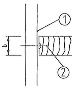
Bild 2 Holzaufleger
