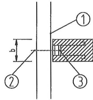
Bild 3 Betonaufleger
