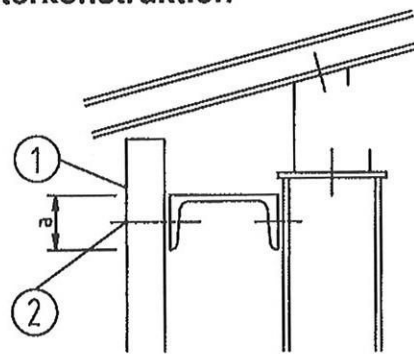
Bild 6 Traufpunkt
