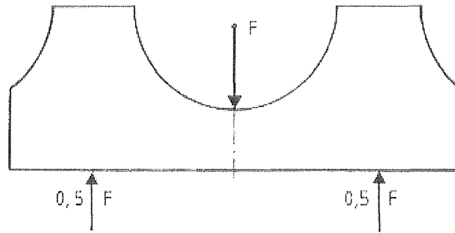
Bild 1: Belastungsanordnung Biegeversuch
