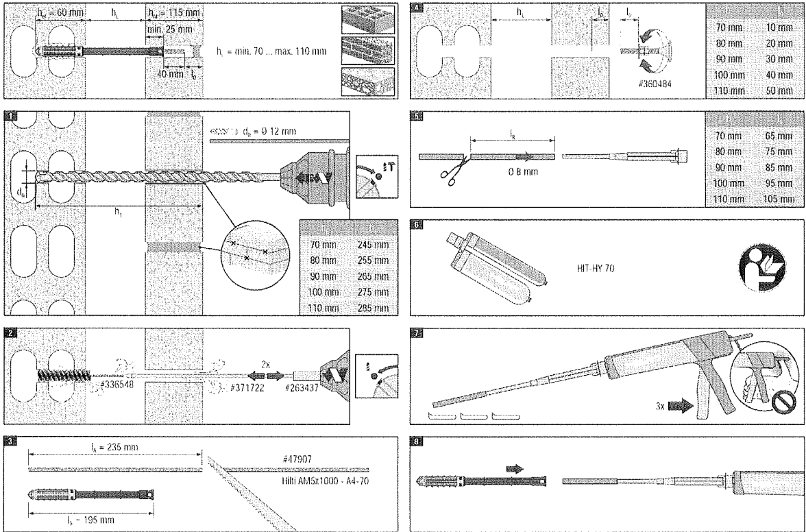
Bild 13: Montageablauf Hilti Mauerwerksvernadelung HIT-MV 70-110
