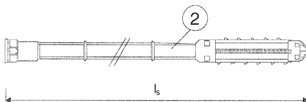
Bild 4: Siebhülselement HIT-MV 0-40, HIT-MV 35-75, HIT-MV 70-110 HIT-MV 110-150 für Schalenabstände 0 \leq h_L \leq 150 \text{ mm}
