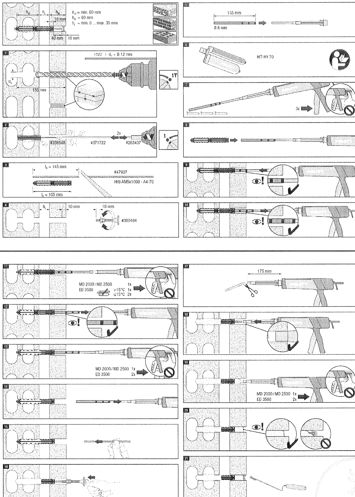
Bild 10: Montageablauf Hilti Mauerwerksvernadelung HIT MV 0-35 (Sparverblender)
