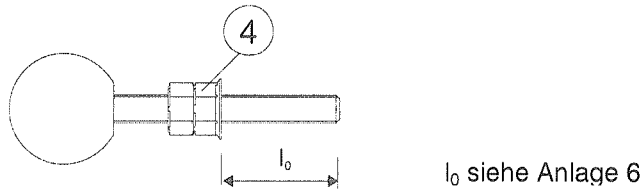
Bild 6: Setzwerkzeug HIT-MVSW zum Einführen der Gewindestange
