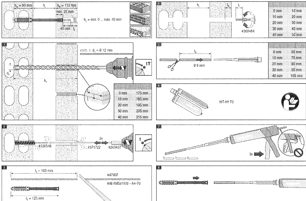
Bild 11: Montageablauf Hilti Mauerwerksvernadelung HIT-MV 0-40
