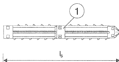
Bild 3: Siebhülselement HIT-MV 0-35 für Sparverblender, Schalenabstände 0 \leq h_L \leq 35 \text{ mm}
